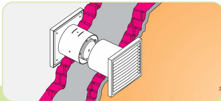
1 – Instalação Kit In-Line 2 – Instalação embutida na parede
